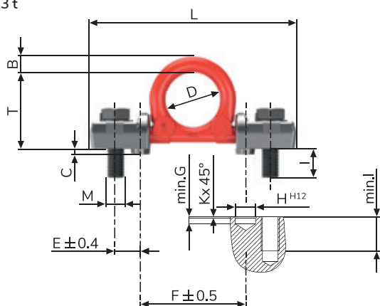
VRBG 10 t / 16 t
