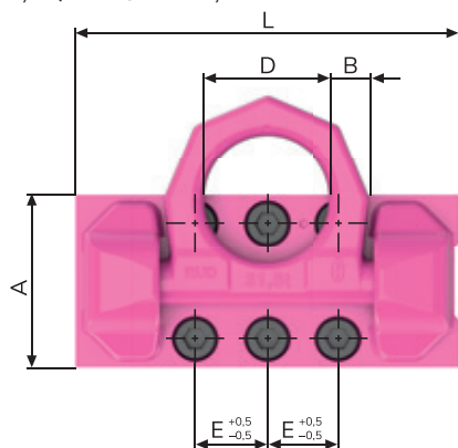
VRBG 31,5 t / VRBG-FIX 31,5 t
