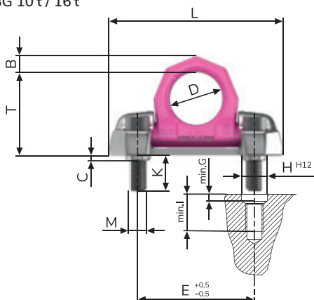
VRBG 10 t / 16 t
