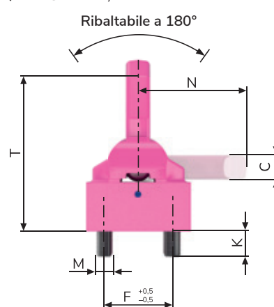
VRBG 31,5 t / VRBG-FIX 31,5 t
