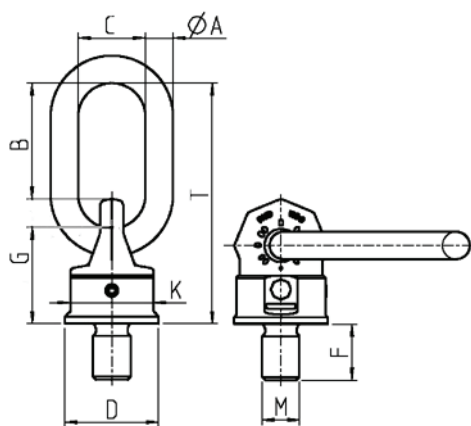
fig. 5: dimensionamento VWBG-Standard
